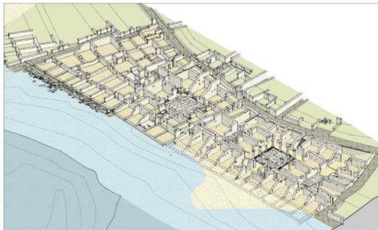
État actuel des vestiges des trois îlots, 1/1000.
